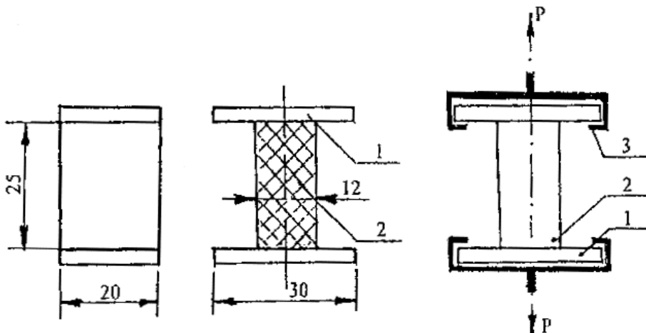
1 - стекло; 2 - герметик; 3 - захват разрывной машины или приспособления
